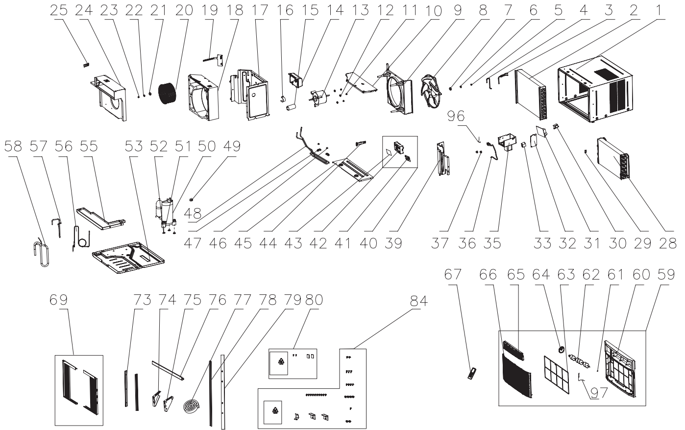
FAM157R1A Parts
