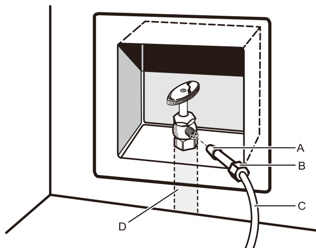
A. Manguito B. Tuerca C. Tubería de cobre (al frigorífico) D. Línea de suministro doméstico
