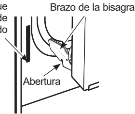
Apoye la abertura en el extremo inferior de la ranura de la bisagra
